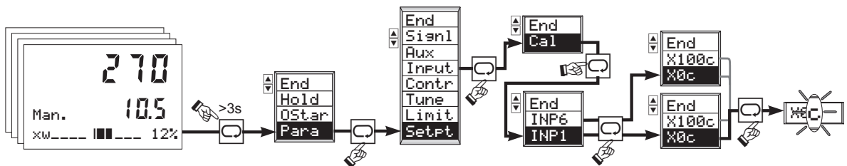
Fig.: 42 Selecting parameter \times 0c / \times 100c
